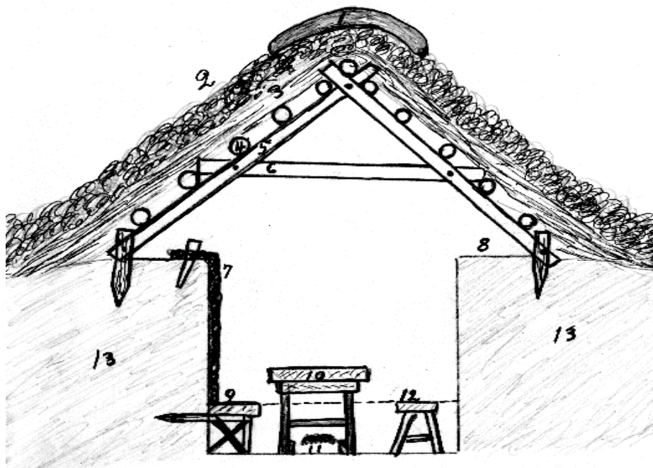
1. Mønningstøv - 2. Lyng - 3. Sogras og hvene - 4. Lægter - 5. Spær af runde rafter - 6. Hanebånd - 7. Græsmatte - 8. På balken havde munken sin plads - 9. Fast bæk - 10. Bord - 11. Her opbevare- des det, som ikke måtte fryse - 12. Løs bæk - 13. Jord
